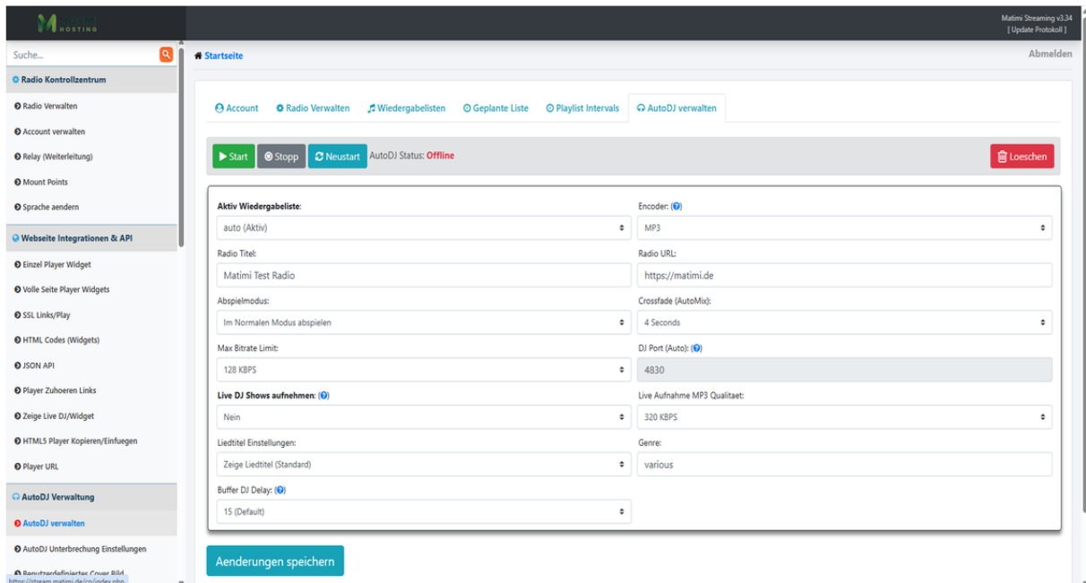
Abbildung 3: AutoDJ-Einstellungen
